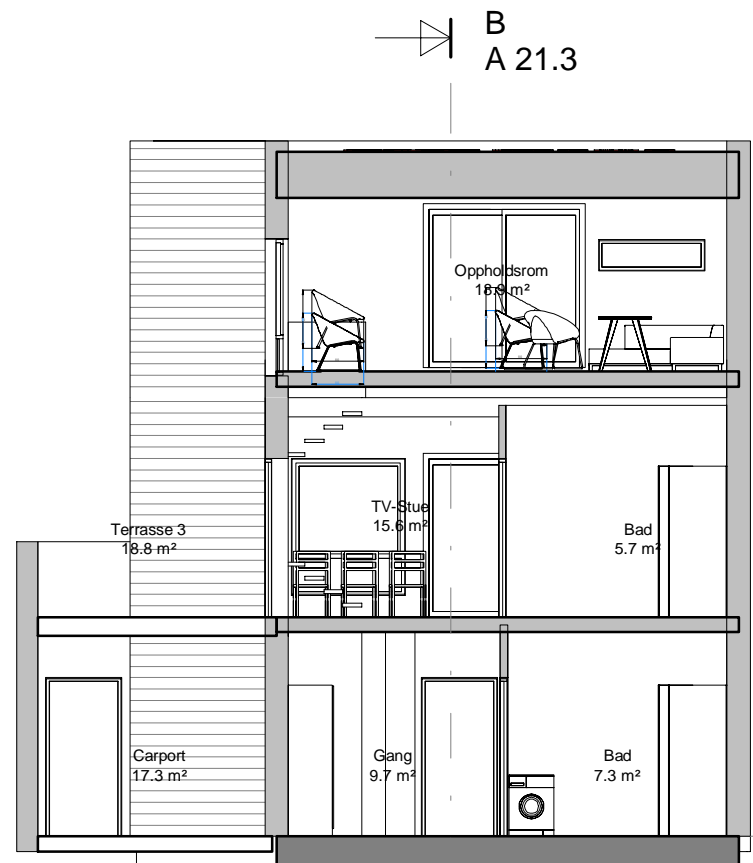
Snitt A-A 1 : 100
