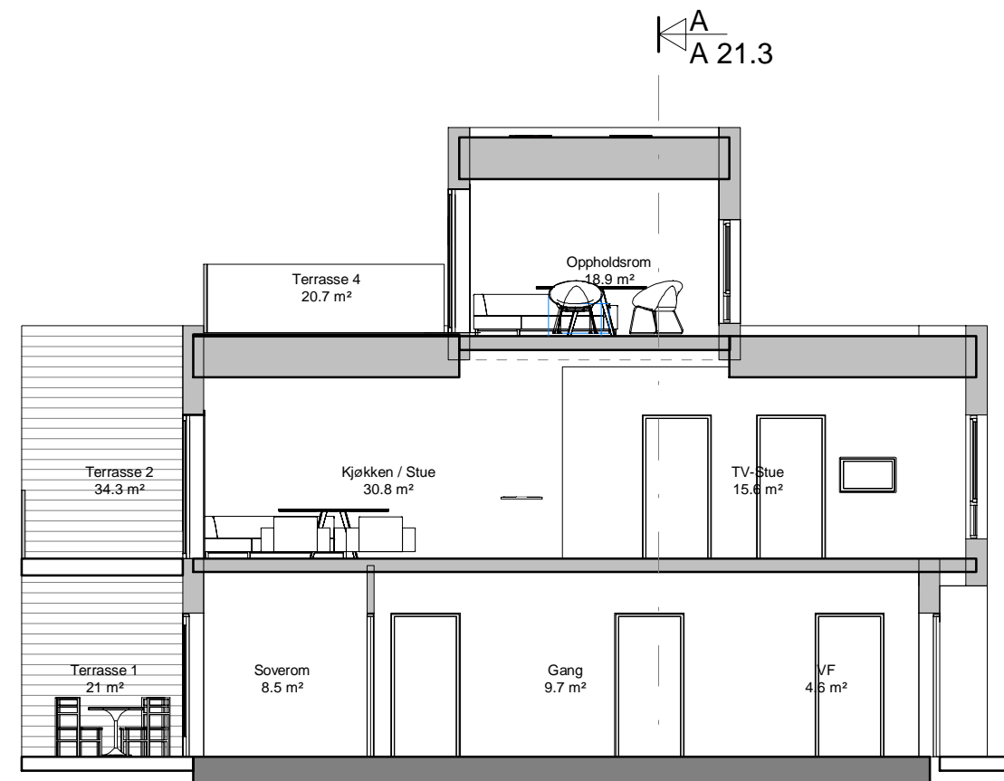
Snitt B-B 1 : 100
