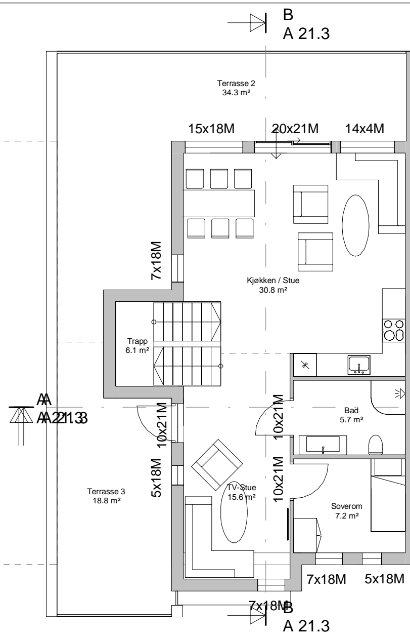
Et. 2 1 : 100
