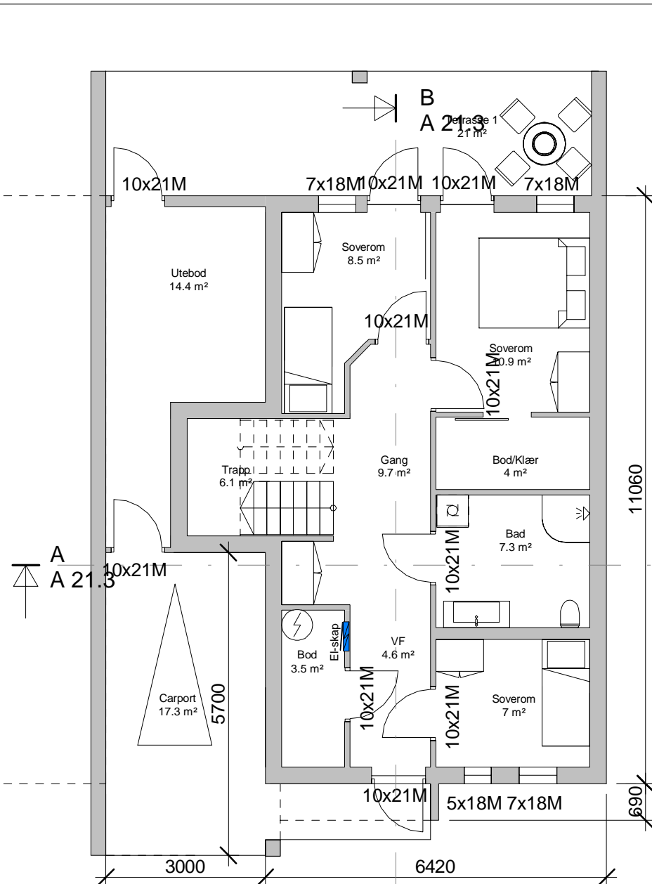
Et. 1 1 : 100
