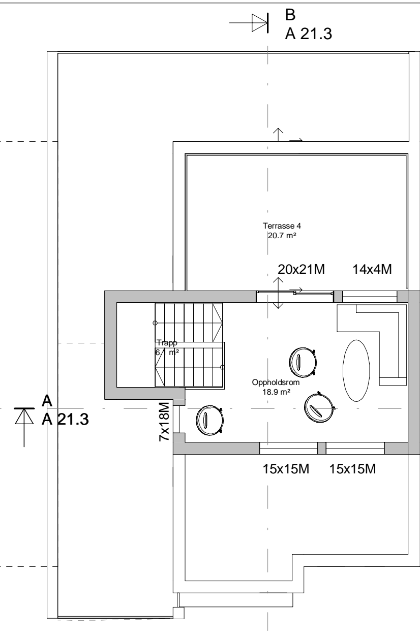
Et. 3 1 : 100
