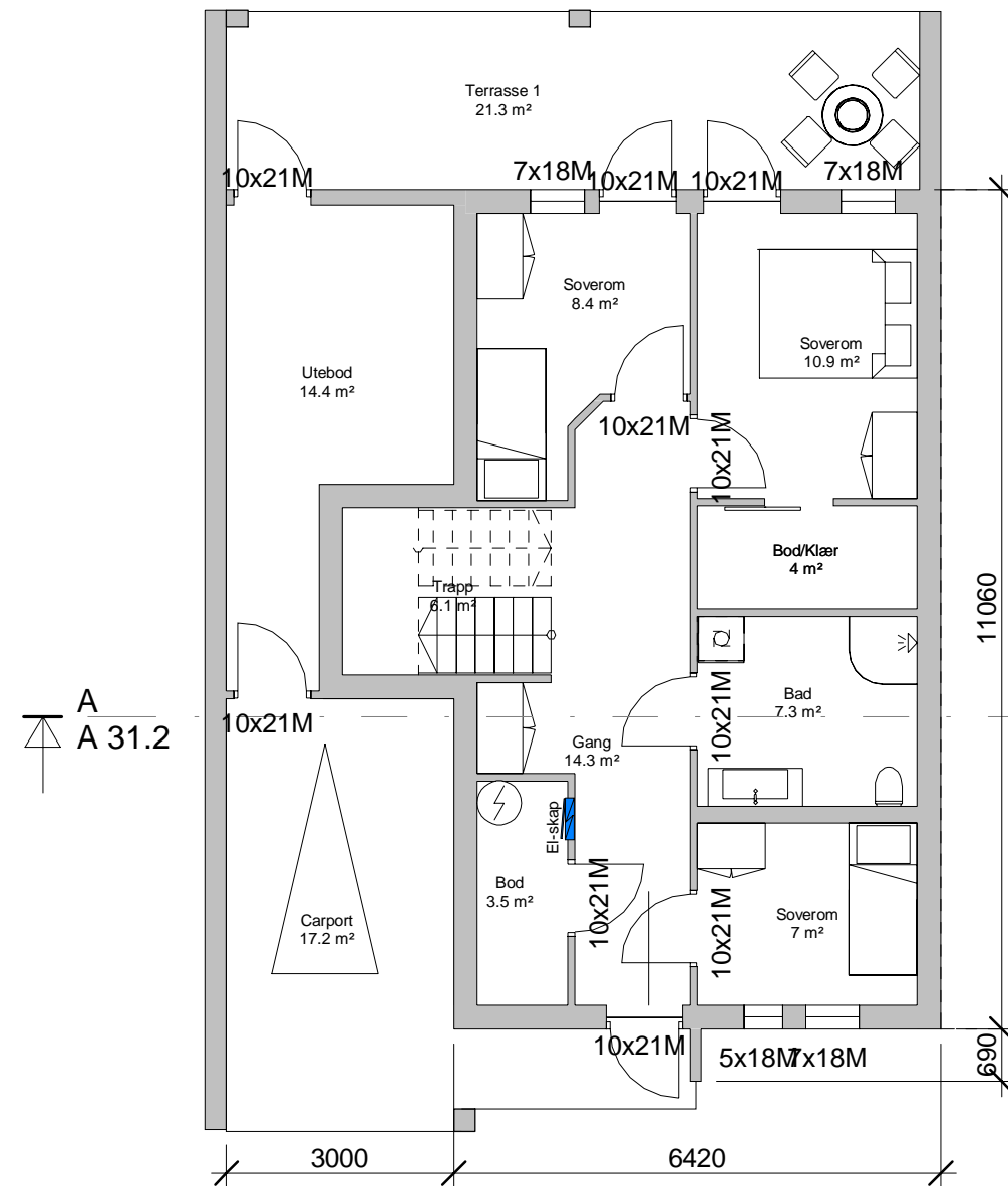
Et. 1 1 : 100
